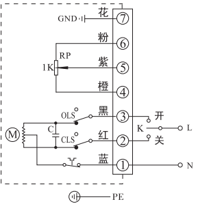
C型：带1KΩ（或500Ω）电位器
