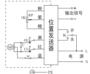
F型：带位置发送器
