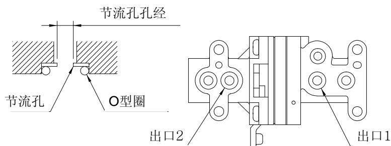
< 节流孔的安装位置和结构 >
