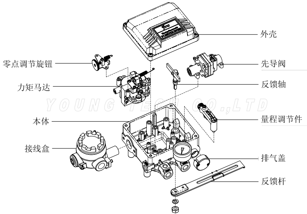
<YT-1000L结构图>
