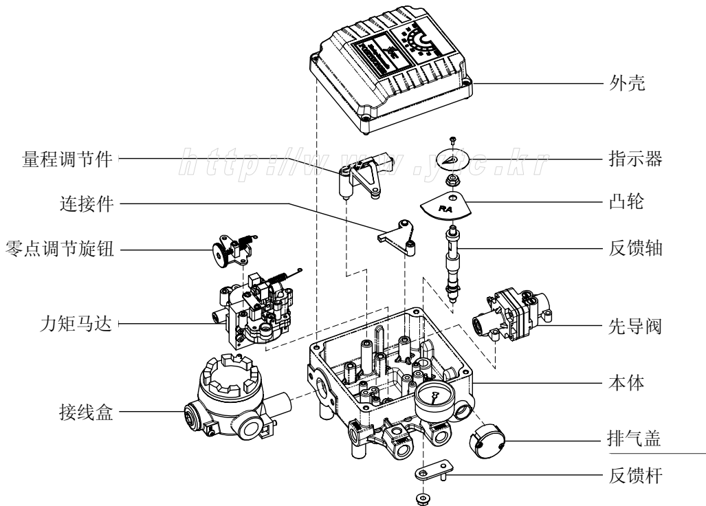
<YT-1000R结构图>
